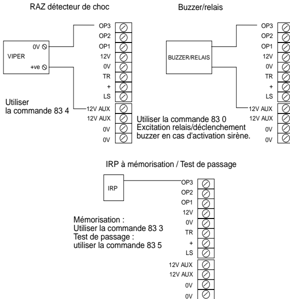
Figure 14. Exemples de câblage pour la sortie programmable OP3
