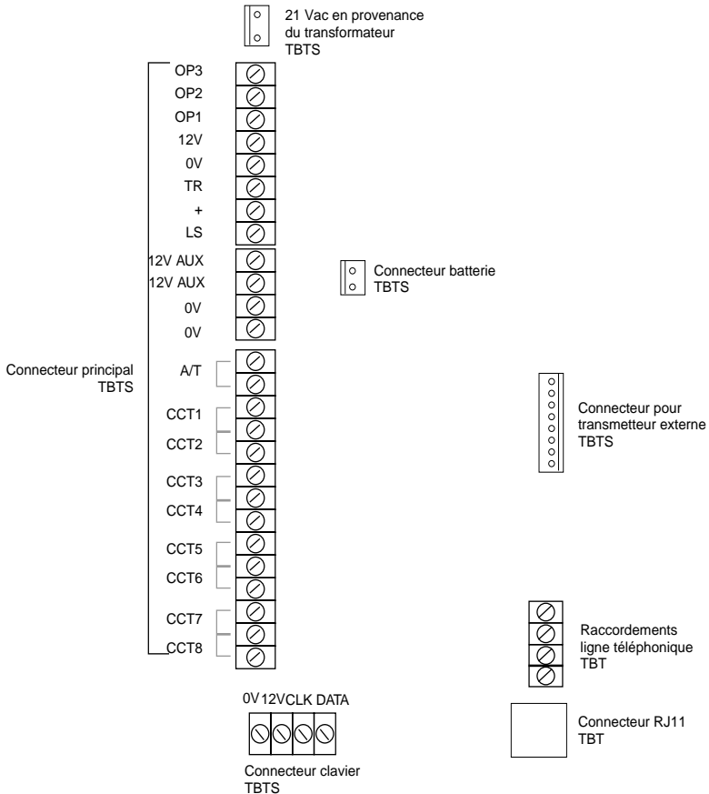
Figure 16. Connecteurs TBT et TBTS de la centrale 9750
