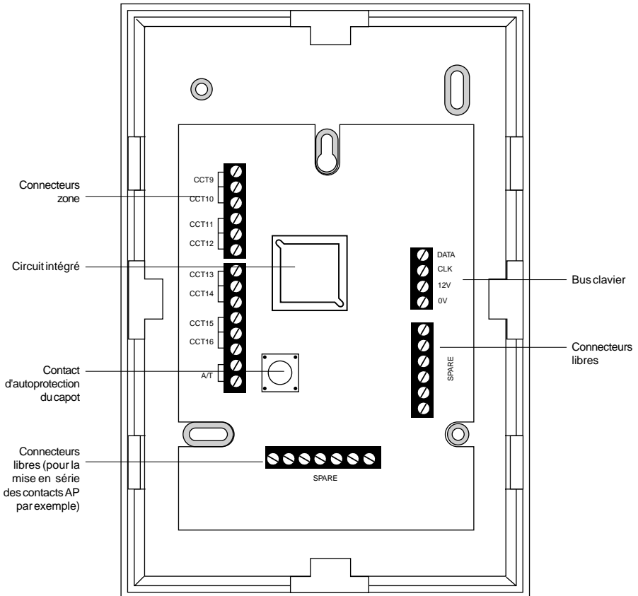
Figure 5. Module d'extension de zones 9755
