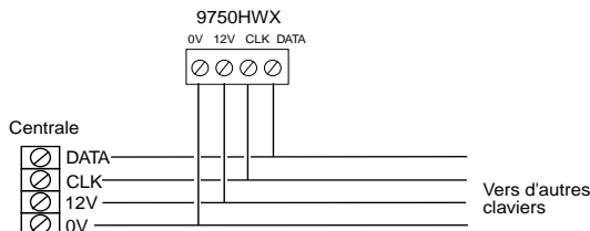
Figure 13. Raccordement d'un module d'extension 9755
