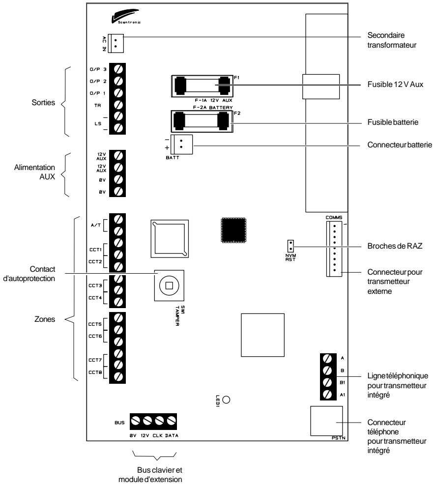
Figure 4. Circuit imprimé de la centrale
