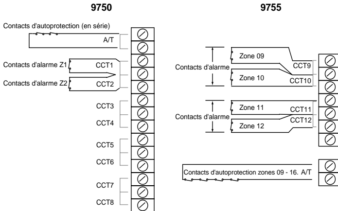
Figure 12. Connexions NF à 4 conducteurs
