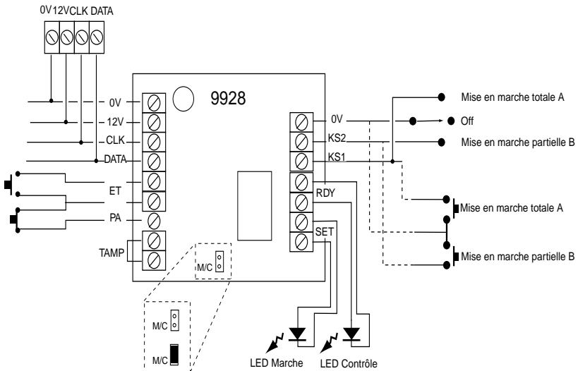
Figure 15. Raccordement d'un boîtier à clé
