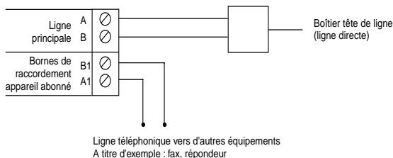
Figure 17. Raccordement du transmetteur intégré
