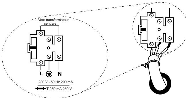
Figure 9. Raccordement secteur
