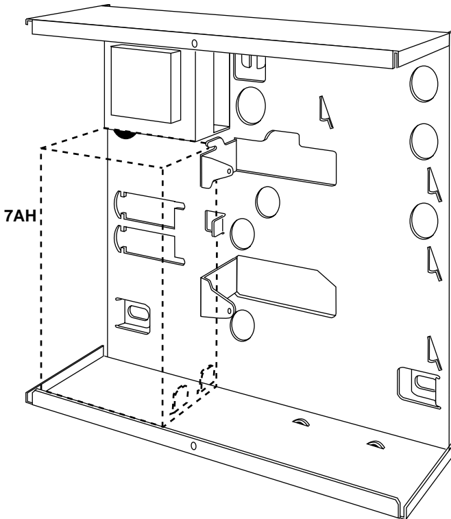
Figure 20. Installation de la batterie
