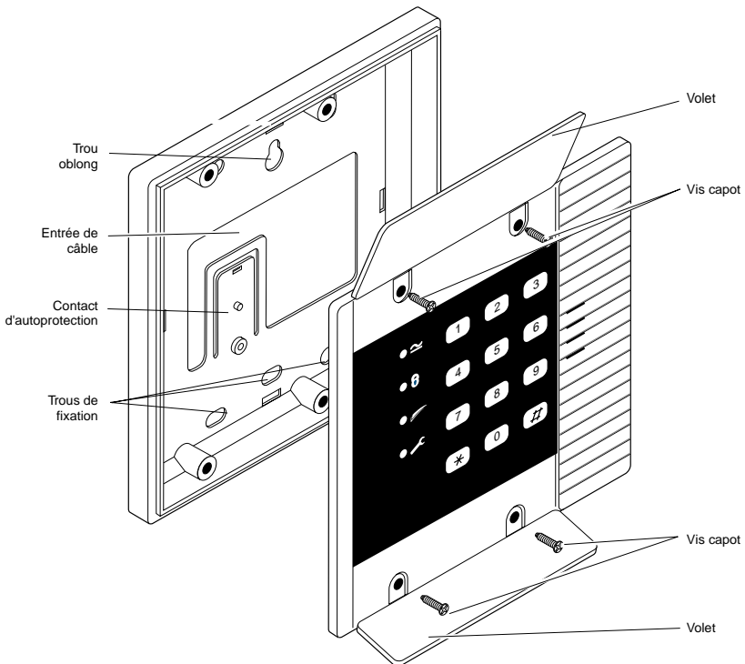
Figure 8. Embase du clavier 9925
