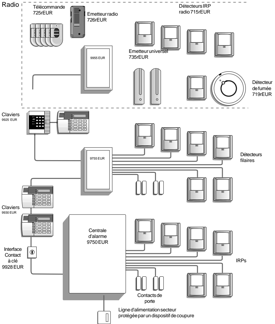
Figure 1. Configuration système 9750
